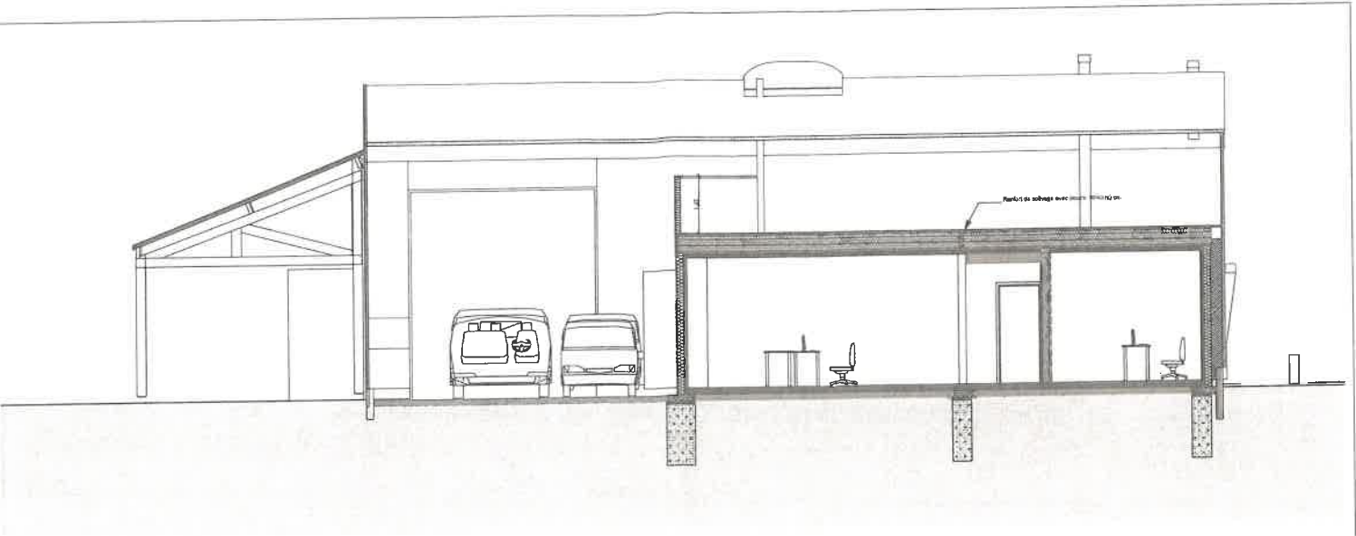
B1 Coupe Transversale
