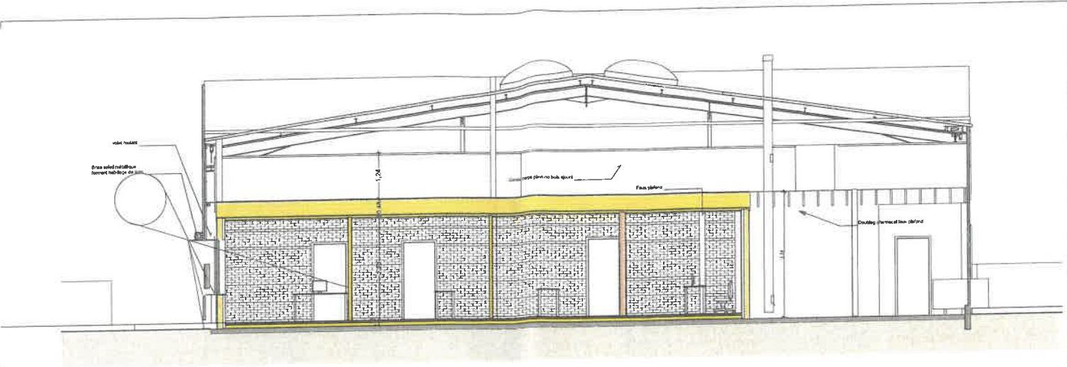
A1 Coupe Longitudinale (1)
